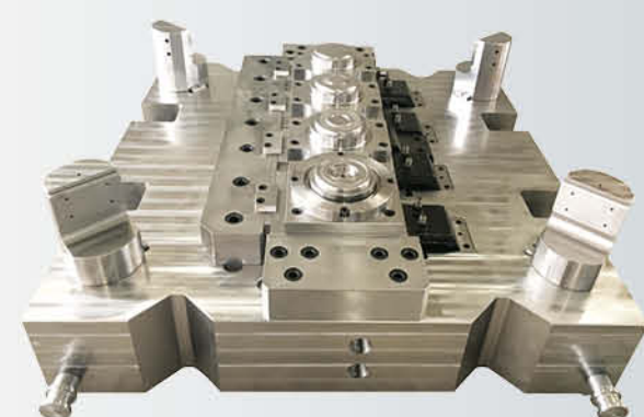
5000T模架
