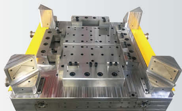
4000T模架
