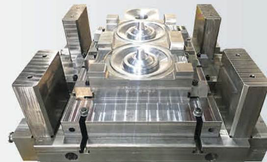
6300T模架
