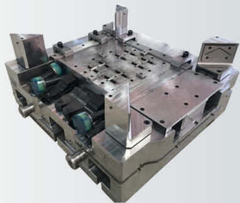
2500T模架
