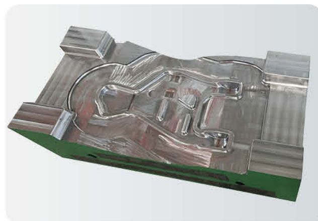
下横臂锻模
