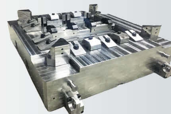
12500T模架
