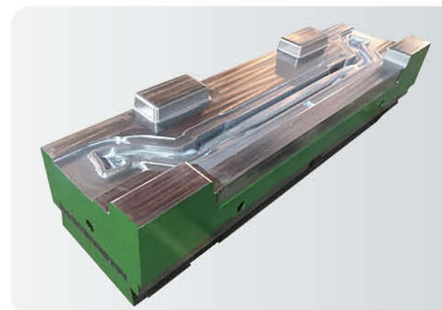
前轴模具
